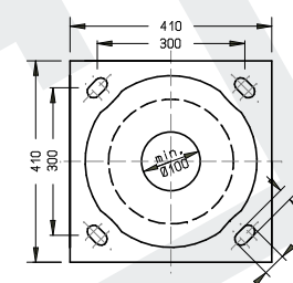
PROPUNERE BULON DE FIXARE STALP CU FLANSA
