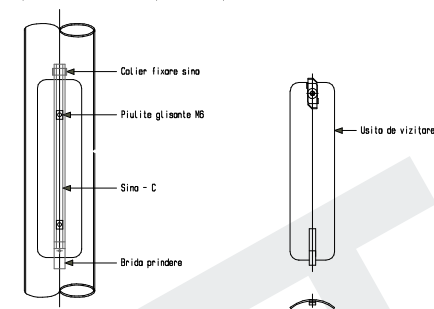
DETALIU A - USITA DE VIZITARE
