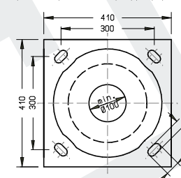
PROPUNERE BULON DE FIXARE STALP CU FLANSA
