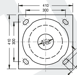
PROPUNERE BULON DE FIXARE STALP CU FLANSA
