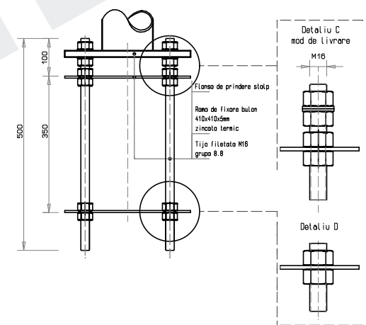
PROPUNERE BULON DE FIXARE STALP CU FLANSA
