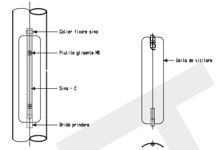
DETALIU A - USITA DE VIZITARE
