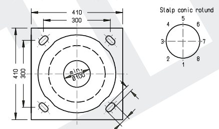
PROPUNERE BULON DE FIXARE STALP CU FLANSA
