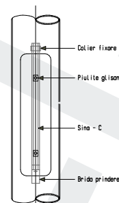
DETALIU A - USITA DE VIZITARE
