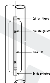
DETALIU A - USITA DE VIZITARE
