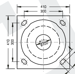
BULON DE FIXARE STALP REFLECTOARE
