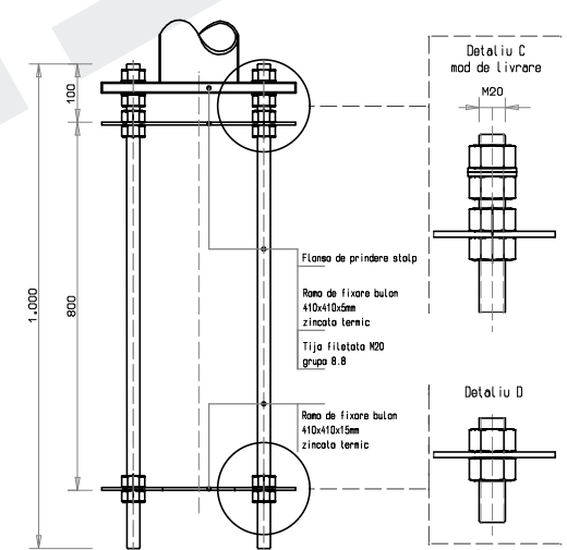
BULON DE FIXARE STALP REFLECTOARE
